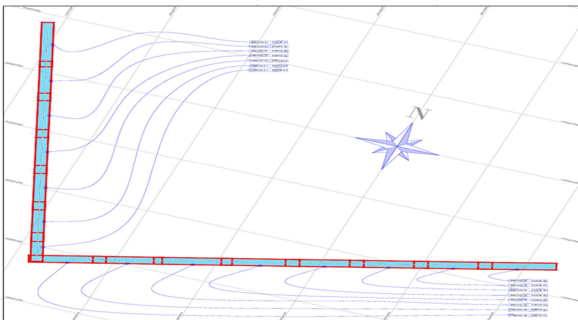
Levantamento topográfico TRECHO 1 .
