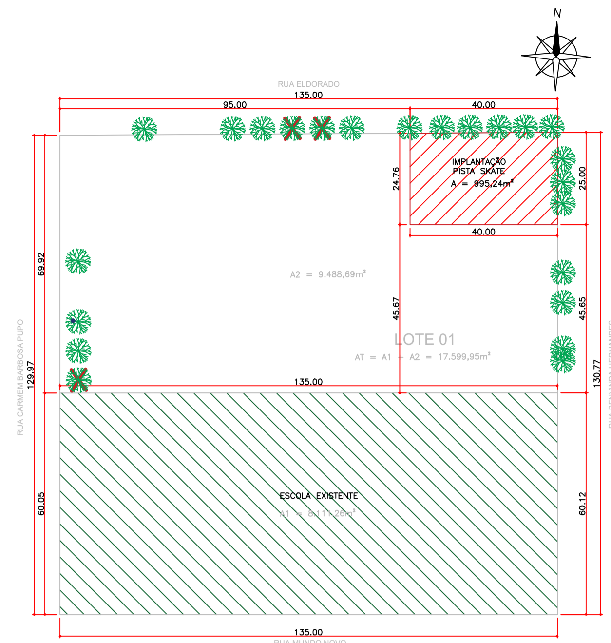
ÁREA DE INTERVENÇÃO PISTA DE SKATE Esc 1:1000
