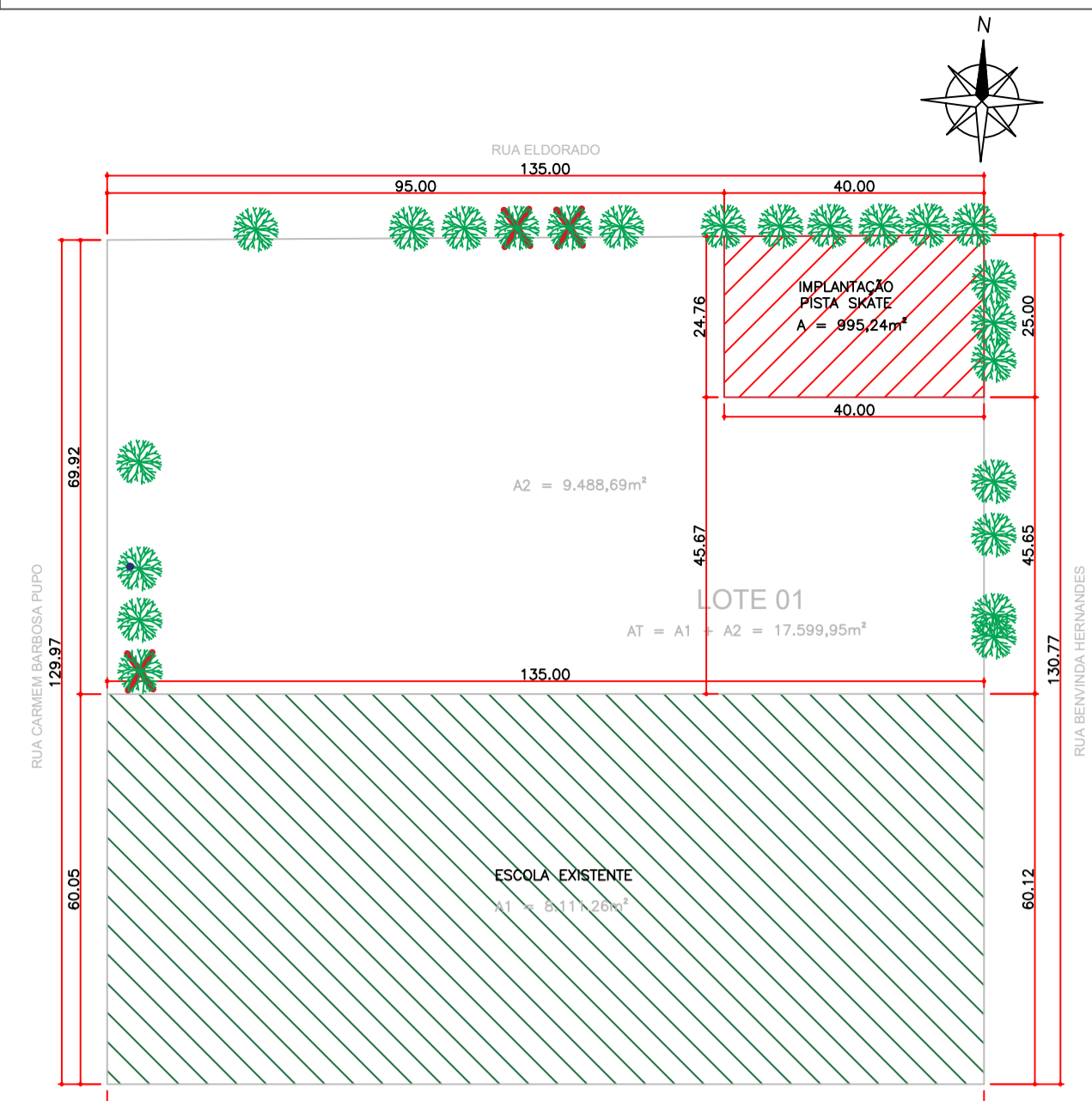
ÁREA DE INTERVENÇÃO PISTA DE SKATE Esc 1:1000
