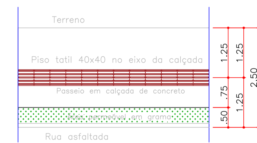
DETALHE DA CALÇADA Sem escala
